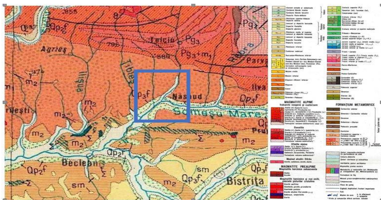
Fig.30. Harta geologică
